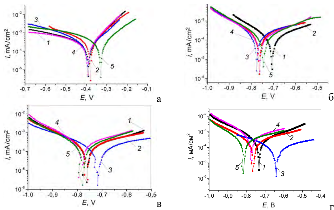
Рисунок 3 – Потенціодинамічні криві напильних електродугових покриттів з порошкових дрітів різного складу: 1 – ПД 90X17P2ГC; 2 – ПД №2 (20X16P3H2ГC); 3 – ПД №3 (90X17PГC); 4 – ПД 90X17P3ГC; 5 – ПД №5 (X17P3C)
