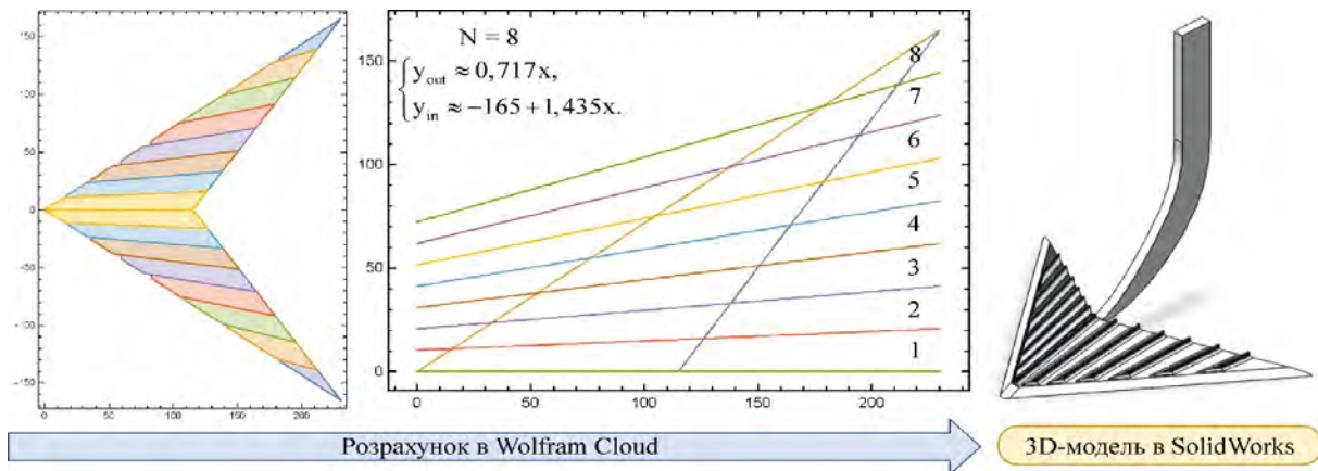
Рисунок 8 – Візуалізація звичайної стрілкової лапи із направляючими променями Джерело: розроблено авторами
