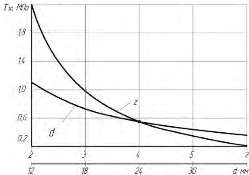
Рисунок 5 – Графічні залежності напружень зрізу \tau_{zp} від кількості пальців z та величини діаметра пальців d при колівій силі F_k=1000 Н
