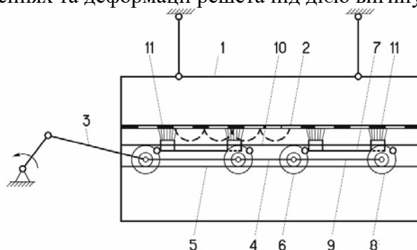
1 – решітний стан; 2 – решето; 3 – привод; 4 – рама; 5 – напрямна; 6, 8 – колеса; 7, 9 – ланки; 10 – опорні доріжки; 11 – щітки
