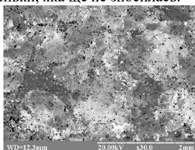
Рисунок 3 – Топографія робочої поверхні сталі 65Г після випробування у середовищі кварцевого піску зернистістю 500 мкм (а) і середовищі карбіду бору В 4 С (б)
