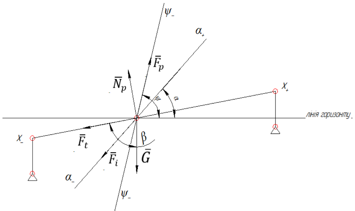
Рисунок 2 – Схема сил, що діють на насінину зернового середовища, яка рухається на поверхні безпротального решета (рух протилежний з напрямом сили інерції) Джерело: розроблено авторами
