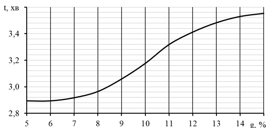
Рисунок 6 – Діаграма для вибору часу змішування при різному вмісті мінімального компонента
