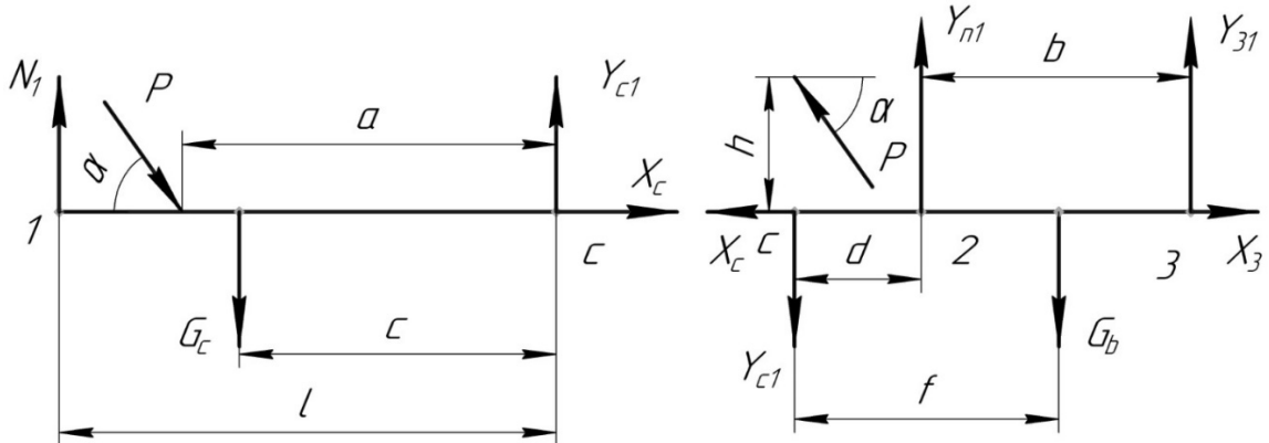
Рисунок 5 – Розрахункова схема до рівняння рівноваги сніці та рами борони МТА (компенсатор зчіпної ваги в режимі навантаження енергетичного засобу та розвантаження борони) Джерело: розроблено авторами
