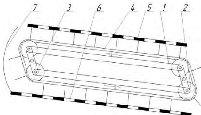
1 – рама; 2–приводний барабан; 3 – натяжний барабан; 4 – полотняно–планчастий транспортер; 5 – верхнє решето; 6 – нижнє решето; 7 – кожух
