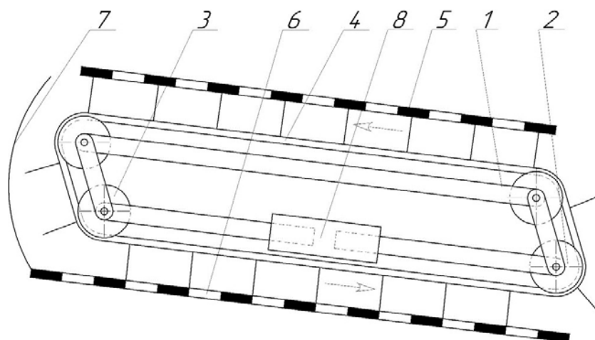
1 – рама; 2–приводний барабан; 3 – натяжний барабан; 4 – полотняно–планчастий транспортер; 5 – верхнє решето; 6 – нижнє решето; 7 – кожух; 8 – механізм регулювання довжини нижньої ланки
