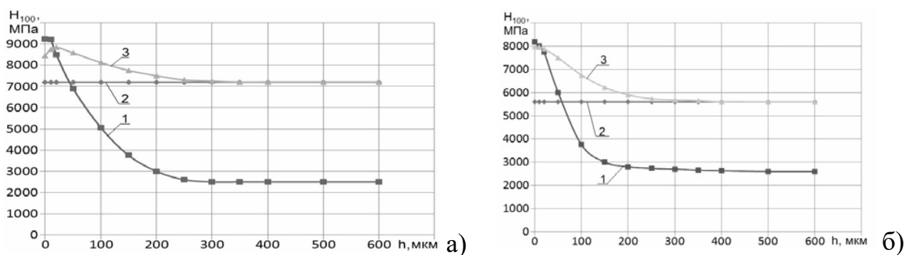
Рисунок 2 – Розподіл мікротвердості від поверхні по глибині титанових сплавів ВТ1-0 (а) і ВТ1-00 (б)
