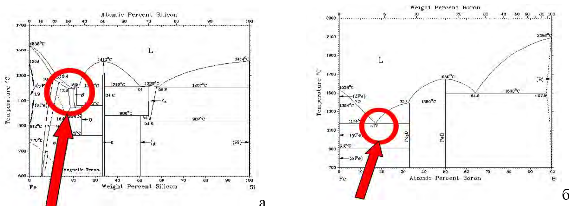
Рисунок 2 - Діаграми стану для заліза та кремнію (а) та заліза й бору (б), що можуть утворювати легкоплавкі евтектики Fe-Si та Fe-B, температура плавлення яких становить відповідно 1212 °C і 1174 °C.
