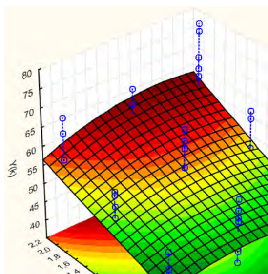
Y = f(x_1x_6)
