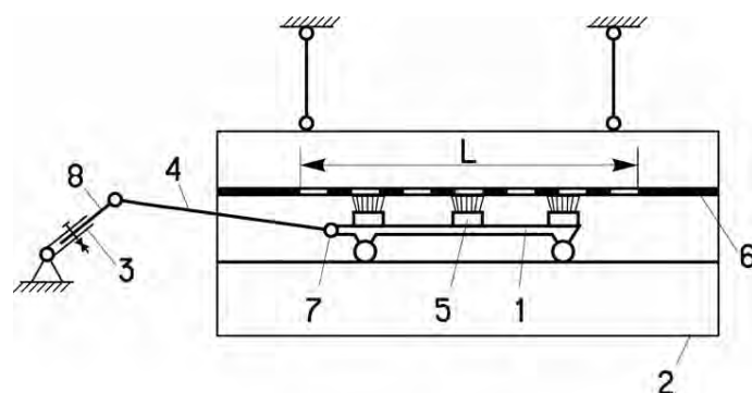
1 – рухома рамка; 2 – решітний стан; 3 – механізм приводу решітного стану; 4 – ведуча ланка; 5 – щітки; 6 – решето; 7 – шарнір; 8 – регулювальна ланка
