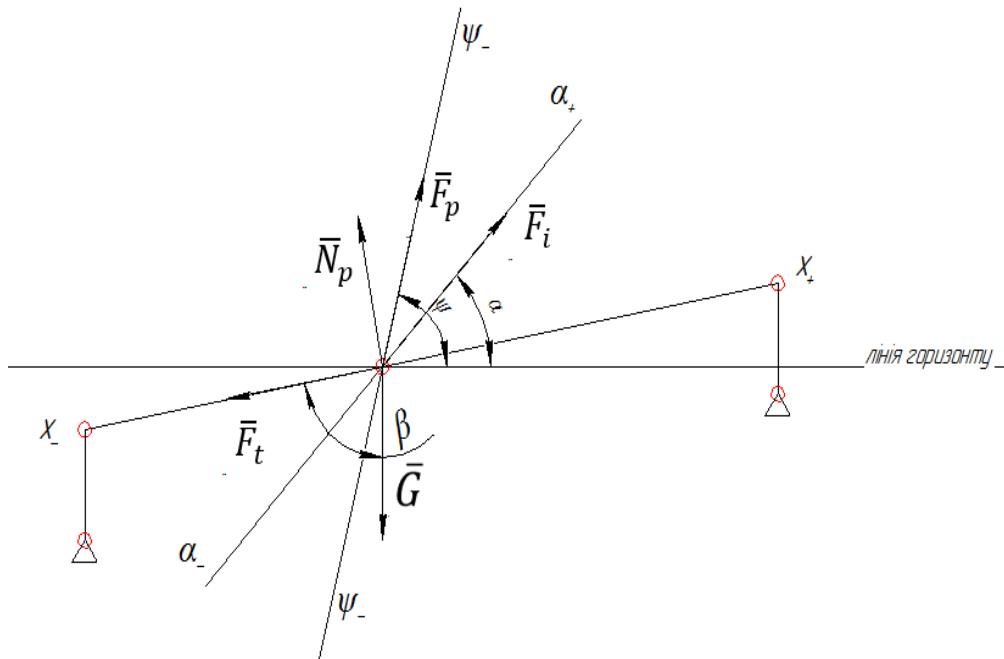
Рисунок 1 – Схема сил, що діють на насінину зернового середовища, яка рухається по поверхні безпротального решета (рух співпадає з напрямом сили інерції) Джерело: розроблено авторами
