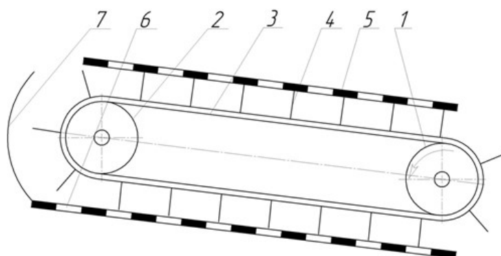
1 – приводний барабан; 2–натяжний барабан; 3 – тяговий елемент; 4 – підпружинені планки;
