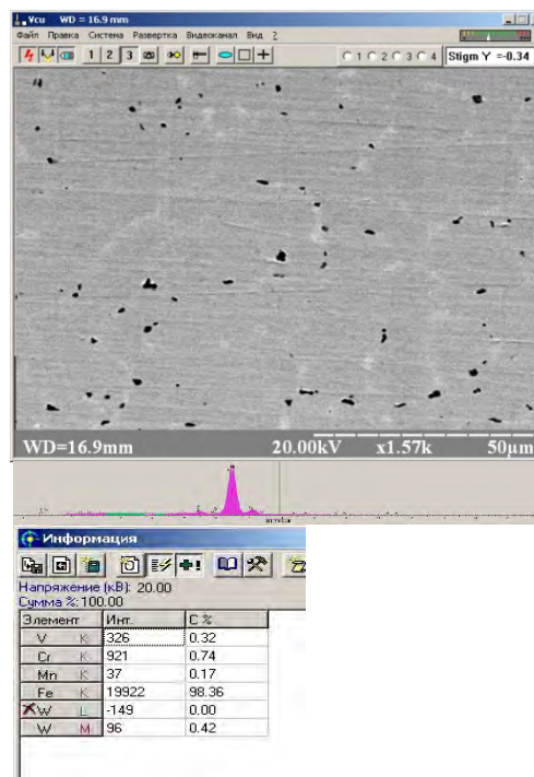
Рисунок 8 – Поверхня тертя молотка дробарки після зміцнення порошковим дротом ПП-АН148 в умовах вільного абразиву, загальна по всій площі перерізу даного покриття Джерело: розроблено автором
