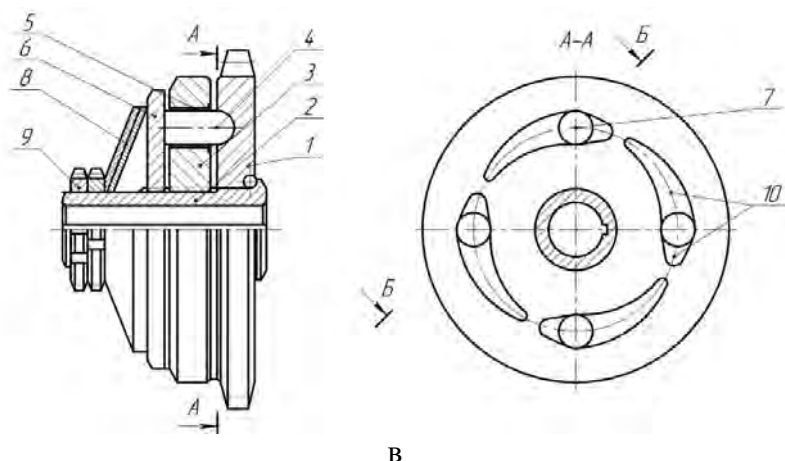
Рисунок 2 – Схема роботи запобіжного пристрою (а) загальний вигляд півмуфти (б) і конструктивна схема запобіжної муфти (в)
