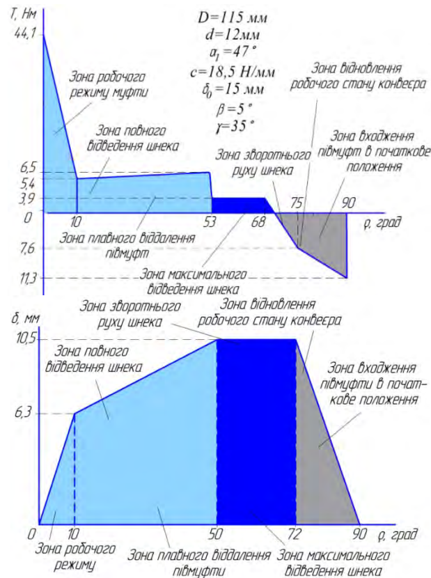
Рисунок 4 – Залежність крутного моменту T (а) та осьового переміщення веденої півмуфти \delta (б) від зміни кута відносного проворотання півмуфти
