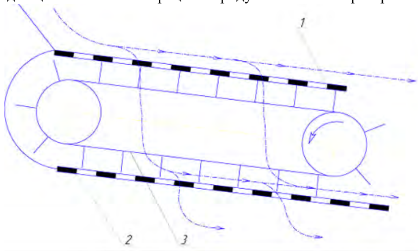
1 – верхнє колосове решето; 2–нижнє підсівне решето; 3 – ланцюгово–скребковий транспортер
