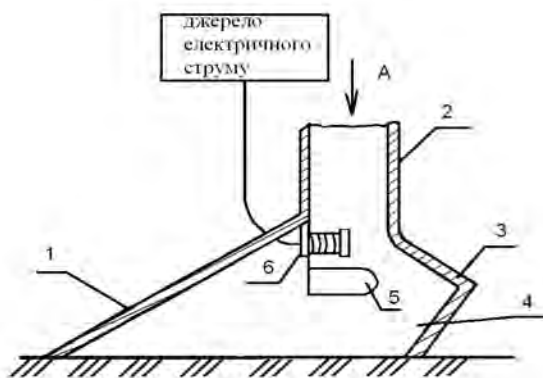
1 – лапа; 2 – насіннєспровід; 3 – щиток; 4 – підлаповий простір; 5 – розподільник; 6 – електромагнітний вібратор
