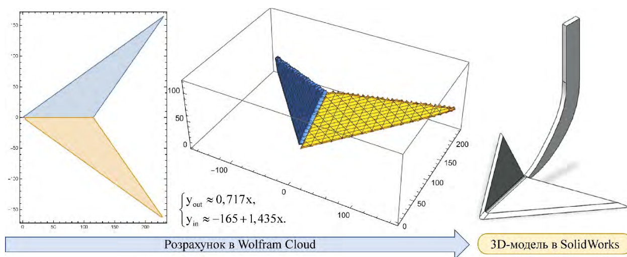
Рисунок 4 – Візуалізація звичайної стрілкової лапи
