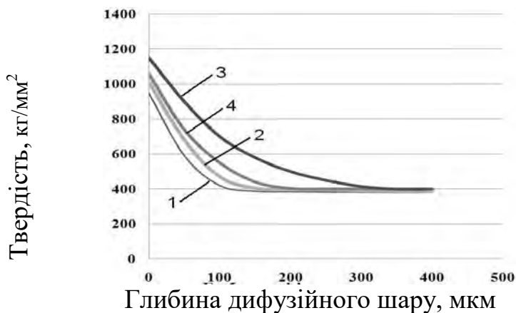
Рисунок 1 – Вплив тривалості циклів на глибину дифузійного шару
