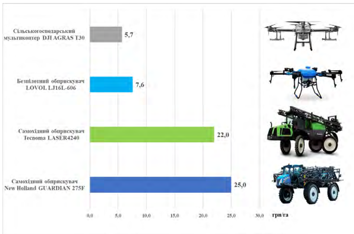
Рисунок 1 – Приведені питомі енерговитрати досліджуваних обприскувачів
