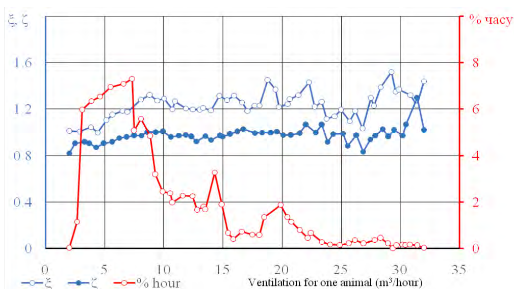
Рисунок 10 – Вплив інтенсивності вентиляції на значення \xi та \zeta в точках автоматичного відбору проб і розподіл частоти інтенсивності вентиляції в приміщенні із системою вентиляції через стінові канали (варіант 3)
