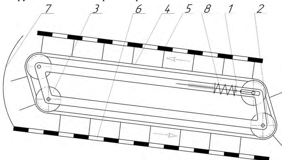
1 – рама; 2 – приводний барабан; 3 – натяжний барабан; 4 – полотняно-планчастий транспортер; 5 – верхнє решето; 6 – нижнє решето; 7 – кожух; 8 – пружинний механізм
