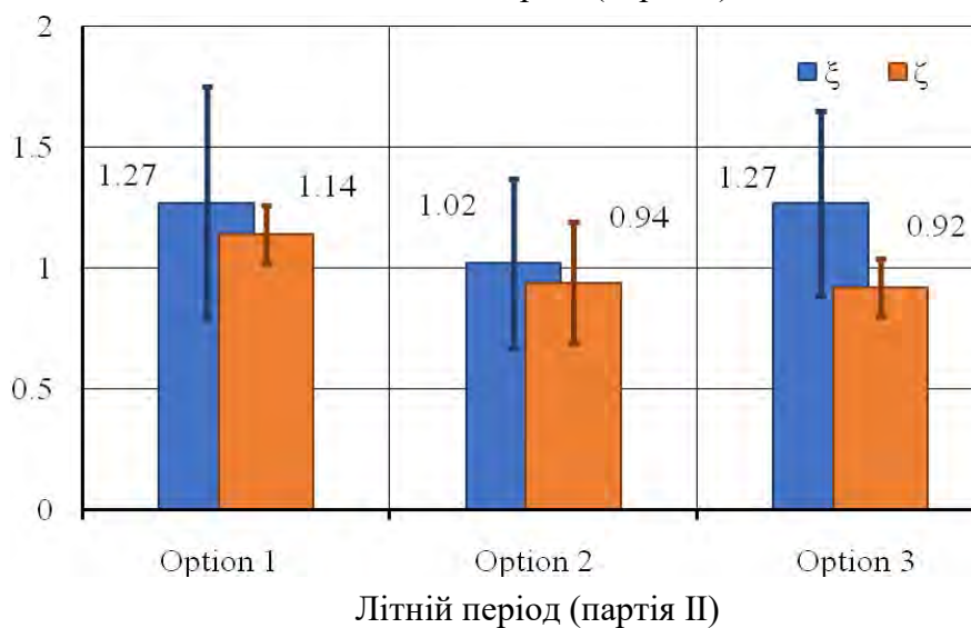
Рисунок 7 – Середні значення ефективності видалення забруднень \xi і ефективності відведення теплоти \zeta з зони перебування тварин
