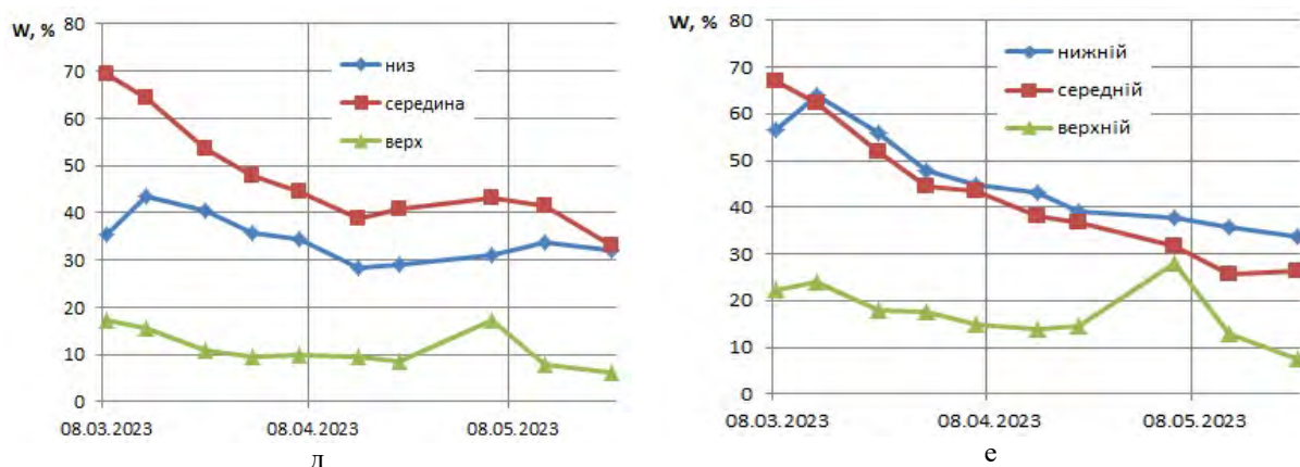
Рисунок 5 – Графічні залежності зміни вологості шарів досліджуваних зразків ґрунту та органічних добрив з часом дослідження для варіантів досліду (табл. 1)
