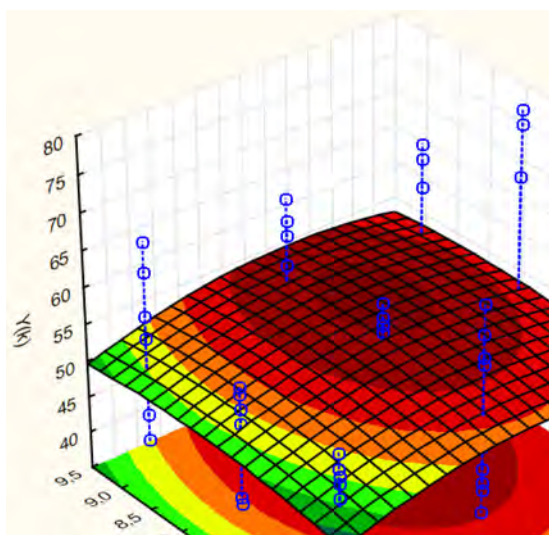
Y = f(x_1x_4)
