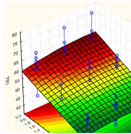
Y = f(x_3x_6)
