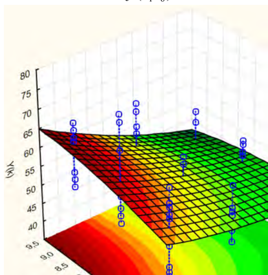
Y = f(x_2x_4)
