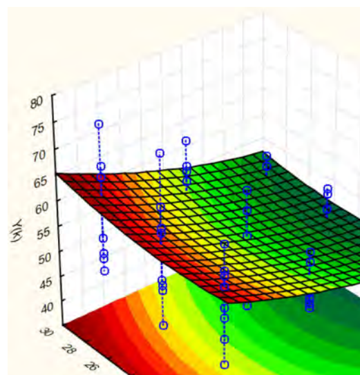
Y = f(x_2x_5)
