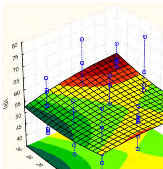
Y = f(x_3x_5)
