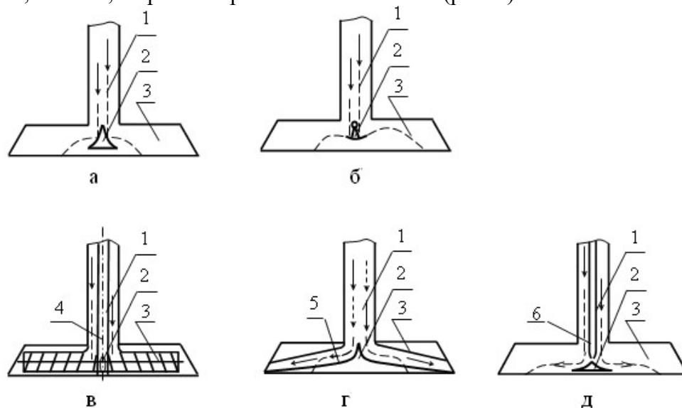
а – з пасивним розподільником; б – з вібраційним розподільником; в – з активним розподільником; г – з пневмотранспортуванням і розсівом; д – з пневморозсівом; 1 – матеріалопровід; 2 – розподільник; 3 – підлаповий простір; 4 – механізм приводу; 5 – горизонтальний канал; 6 пневмопровод; ———— – матеріал, що висівається, ———— – повітря
