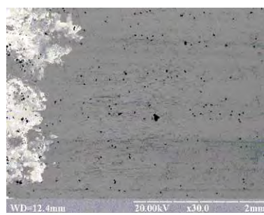
Рисунок 3 – Топографія робочої поверхні сталі 65Г після випробування у середовищі кварцевого піску зернистістю 500 мкм (а) і середовищі карбіду бору В 4 С (б)
